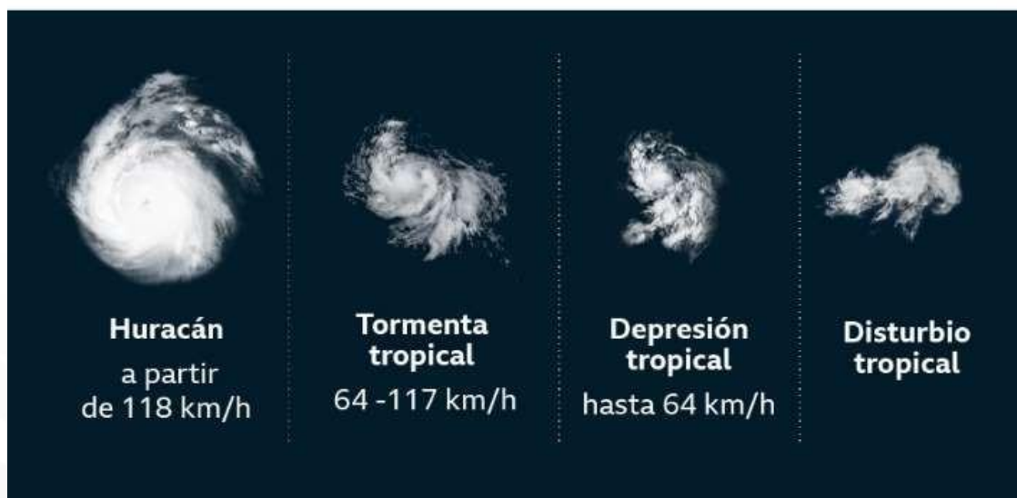
Ilustración 1: Génesis de un sistema tropical.
